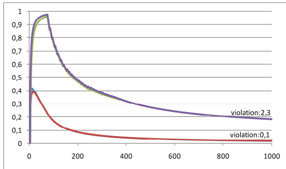
Fig. 10. Viol. cum. avg. (%) for BCT (d) and BestPathMinimax
