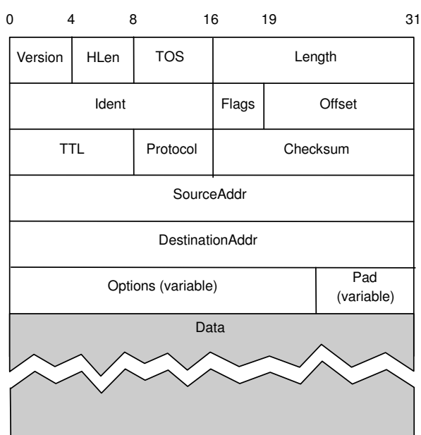
IPv4
